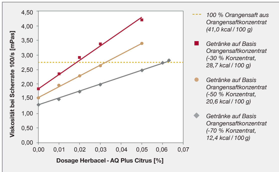
Abb. 2: Abhängigkeit der Viskosität von der Dosage Herbacel - AQ Plus Citrus in Getränken auf Basis Orangensaftkonzentrat
