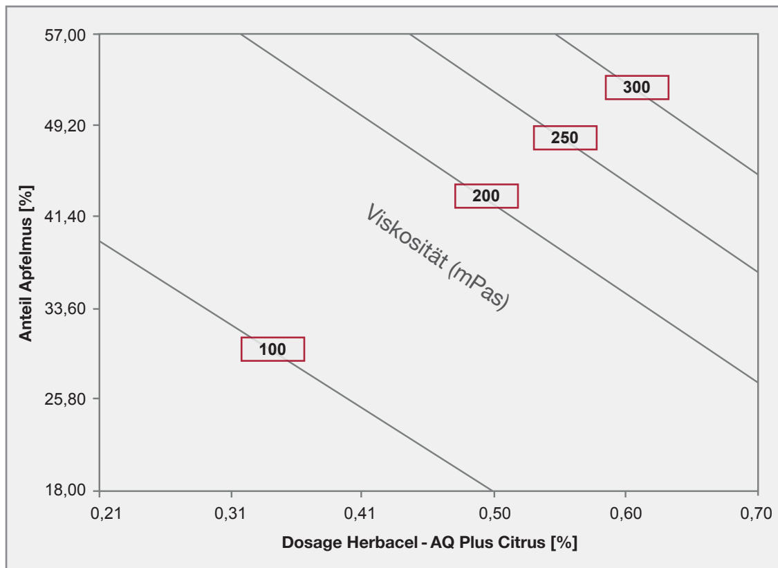
Abb. 3: Viskositätseinstellung eines Fruchtmuses, bestehend aus Apfelmus und Wasser, durch den Einsatz von Herbacel -AQ Plus Citrus
